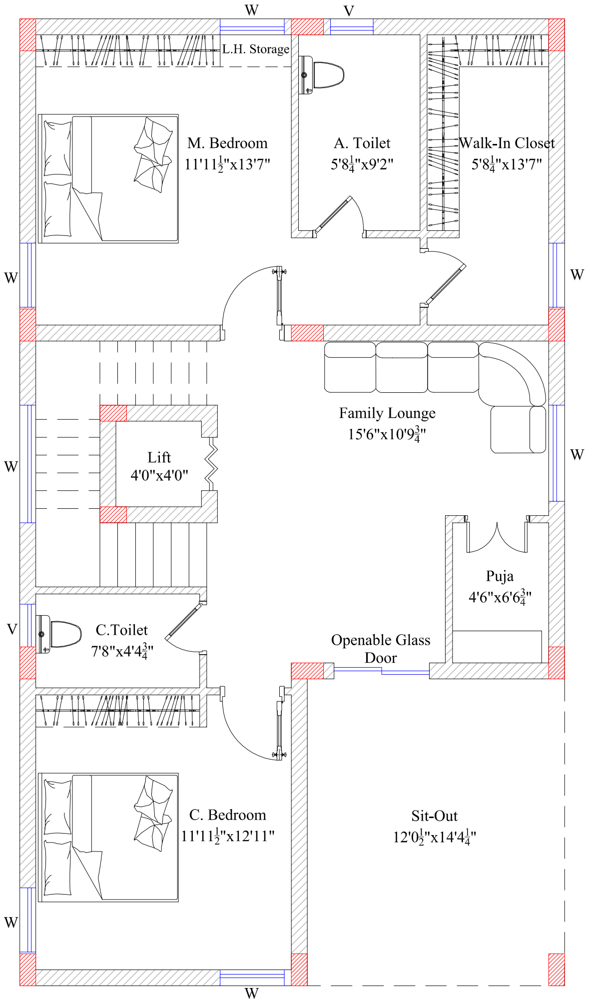
F.F Plan
